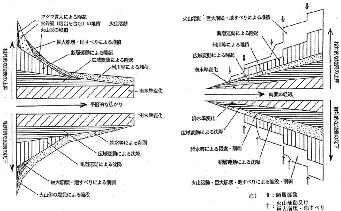
図1 地殻の変動の平面的な広がりや年代的な経過
